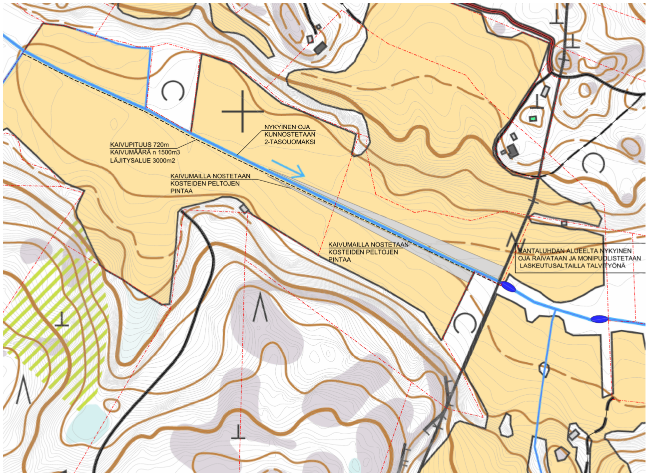
Kuva 1: Kirvunoja muutetaan 720 metrin matkalta kaksitasouomaksi.
